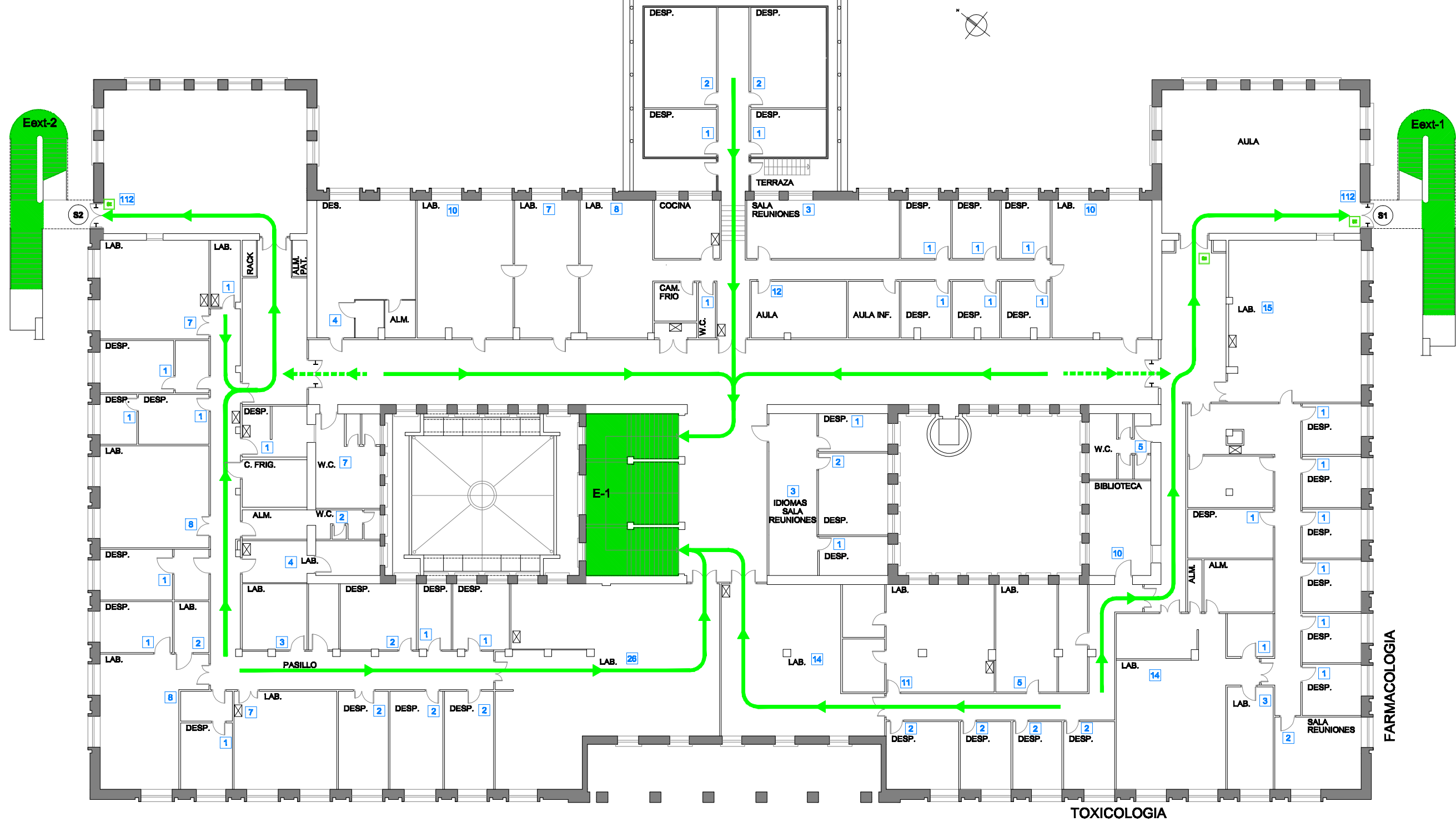
PLANTA PRIMERA OCUPACION MAX.: 485 personas
