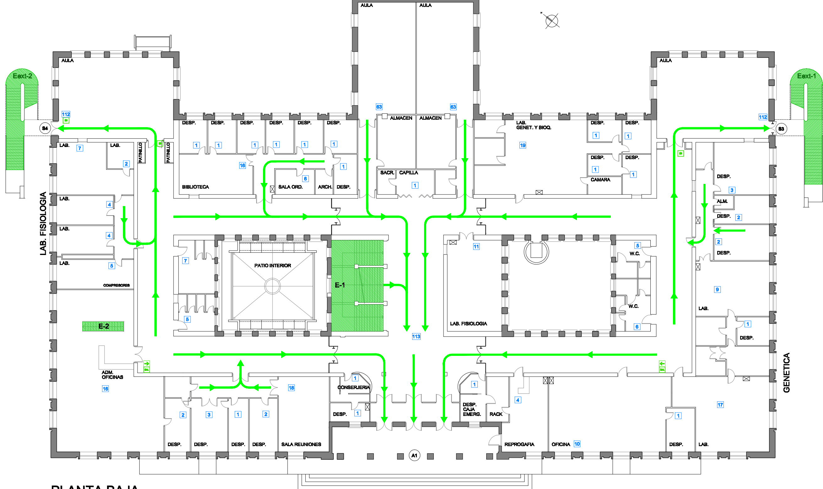
PLANTA BAJA OCUPACION MAX.: 667 personas
