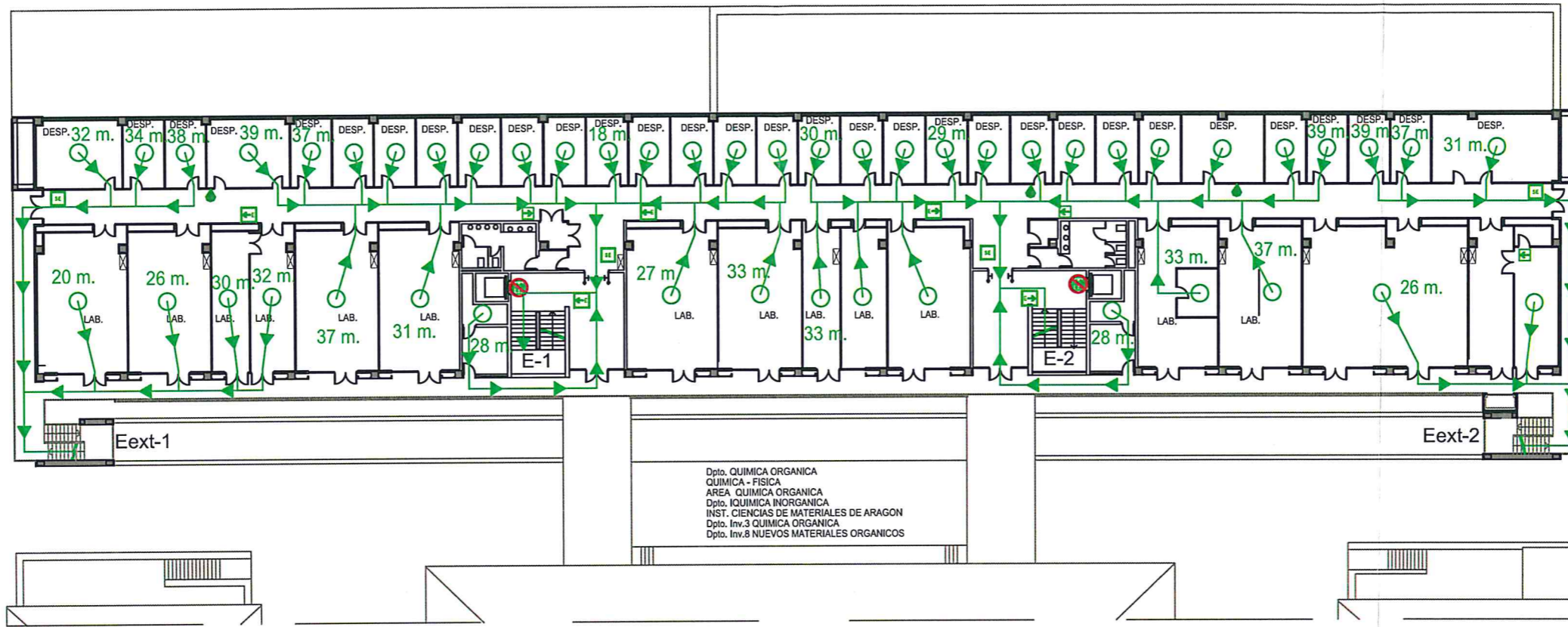
PLANTA TERCERA
