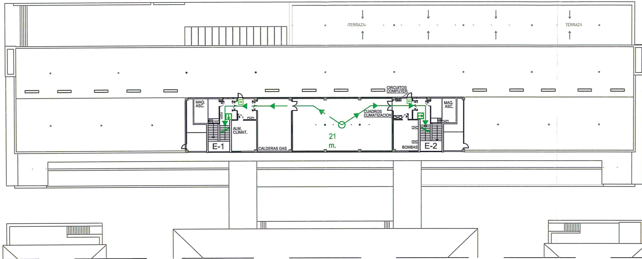
PLANTA DE CUBIERTA
